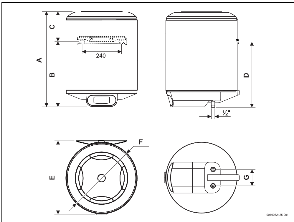
Сл. 2 Димензии во мм (закачено на сид, вертикален склоп)
