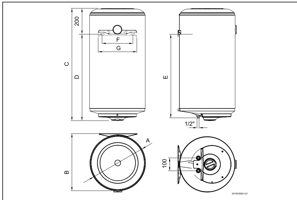
2. ábra Méretek mm-ben (falra szerelés, független szerelés)
