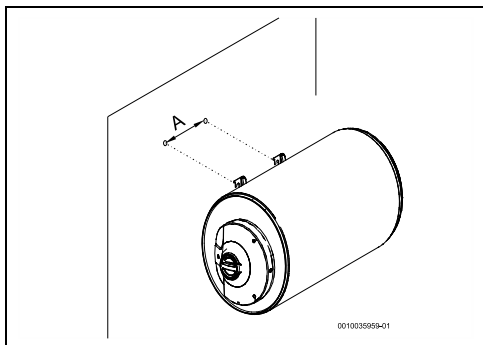
Sl.11 Horizontalna instalacija (pričvršćivanje na zid, TR1000...H)
