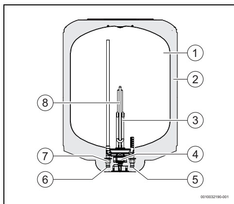
Rys. 4 Komponenty urządzenia
