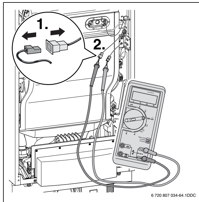
Fig. 48 Racordul multimetrului
