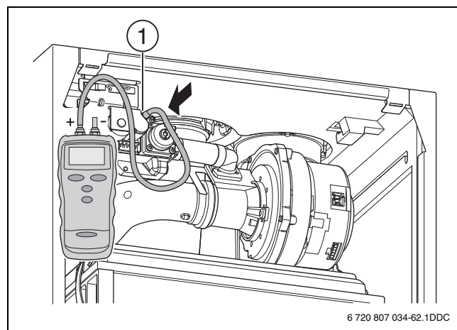
Fig. 43 Racord al manometrului la tip 70
