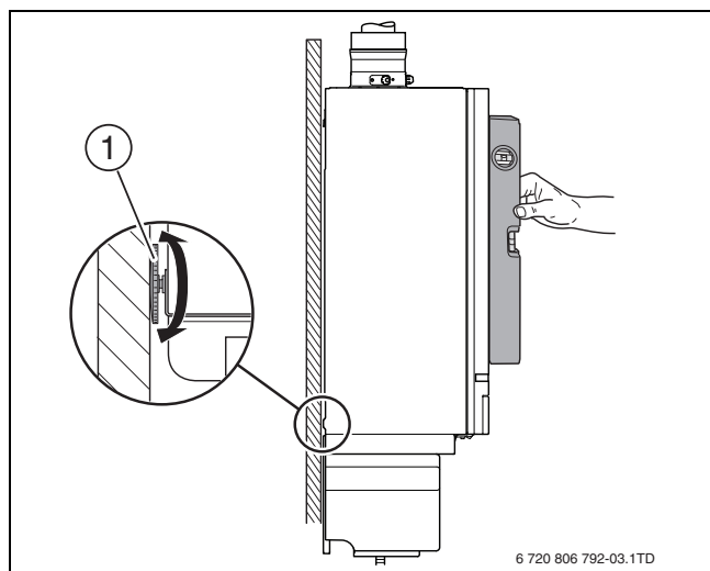
Fig. 11 Poziționarea recuperatorului de căldură cu gaz
