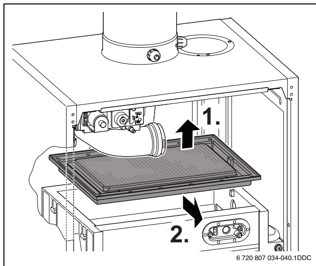
Fig. 56 Îndepărtarea arzătorului
