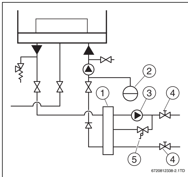
Fig. 17 Montarea buteliei de egalizare hidraulică
