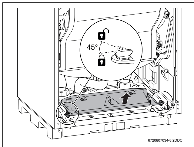
Fig. 26 Îndepărtarea aparătoarei
