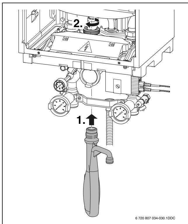
Fig. 19 Montarea sifonului pentru condensat
