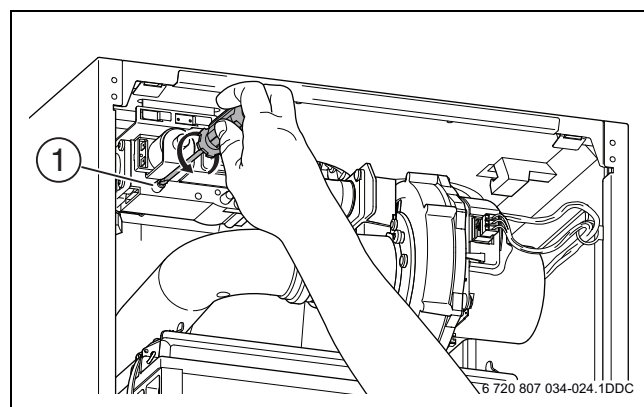
Fig. 42 Deschiderea niplului de presiune de ardere la tip 100
