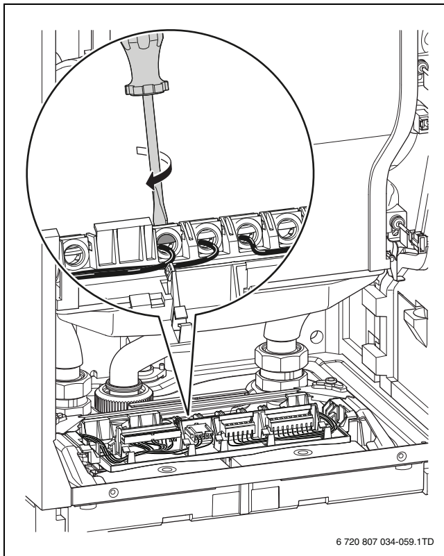
Fig. 29 Strângerea șurubului
