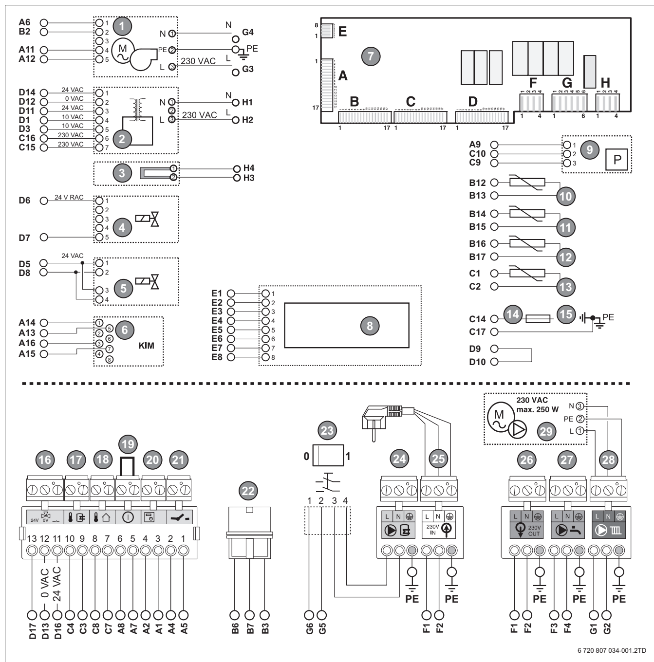
Fig. 5 Schemă electrică
