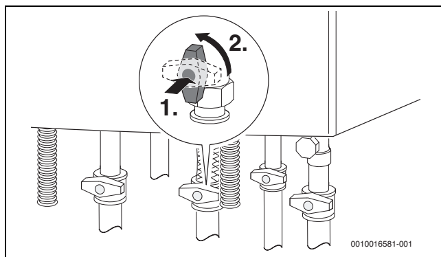
Fig. 3 Deschiderea robinetului de gaz
