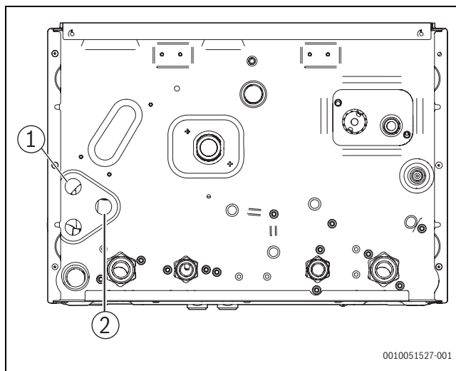
Fig. 34 Diametru cablu
