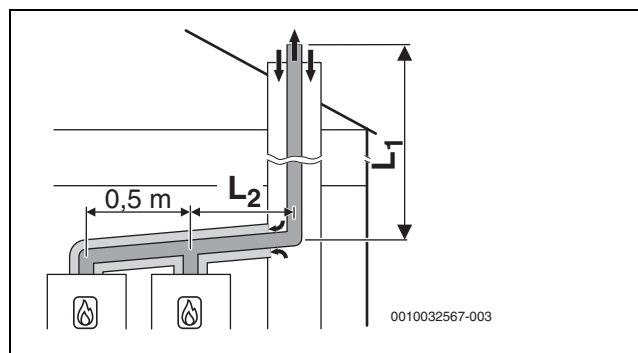
Fig. 28 Cascadă cu 2 aparate:
