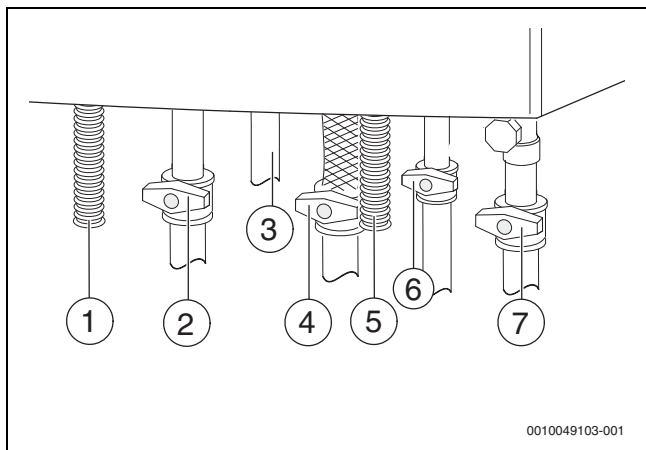
Fig. 32 Racorduri pe partea de gaz și apă (accesorii)
