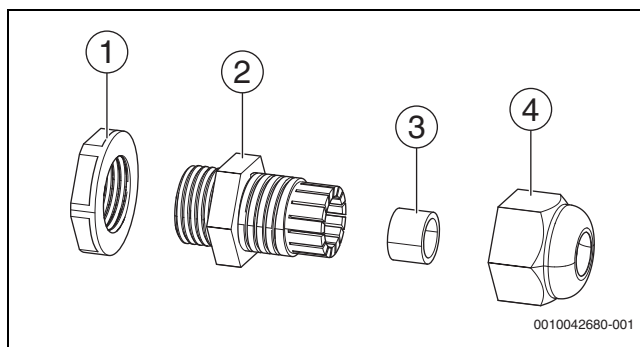
Fig. 35 Piese înfiletare cablu
