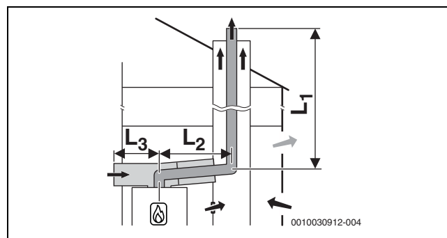
Fig. 11 Ghidarea rigidă a gazelor arse în puț conform C 53x și ghidarea aerului/gazelor arse cu alimentare cu aer separată și evacuare concentrică a gazelor arse în încăpărea centralei termice
