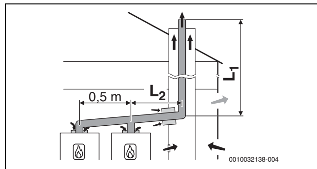
Fig. 27 Cascadă cu 2 aparate: Ghidarea rigidă a gazelor arse în puț conform B 53p cu alimentare cu aer dependentă de aerul din incintă la nivelul aparatului și tubulatură pentru gaze arse cu un perete în încăperea centralei termice; aerisire posterioară în puț
