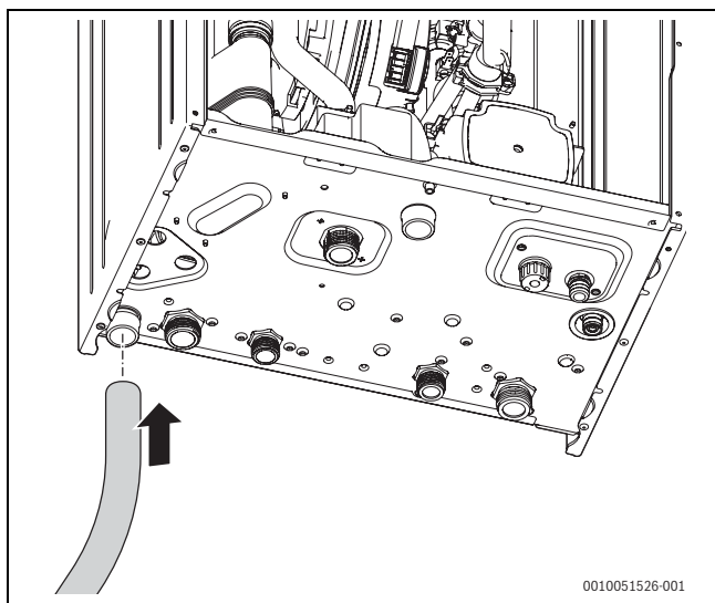
Fig. 31 Montarea furtunului la sifonul pentru condensat
