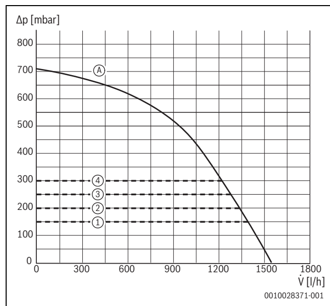
Fig. 153 Câmpuri caracteristice ale pompei și linie caracteristică a pompei (17/24 kW)
