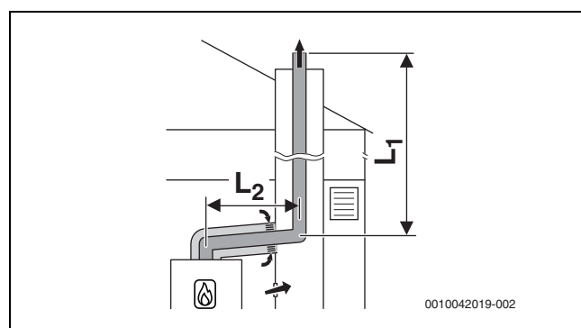
Fig. 32 Ghidarea rigidă a gazelor arse în puț conform B 53p cu alimentare cu aer dependentă de aerul din încălț prin ghidarea concentrică a aerului/gazelor arse în încăperea centralei termice
