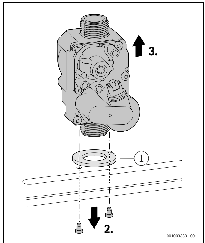
Fig. 138 Demontarea vanei de gaz
