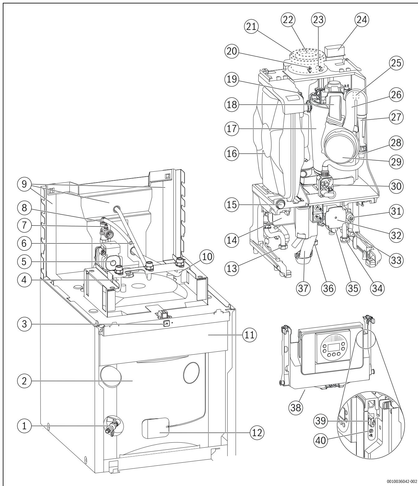
Fig. 5 Structura echipamentului
