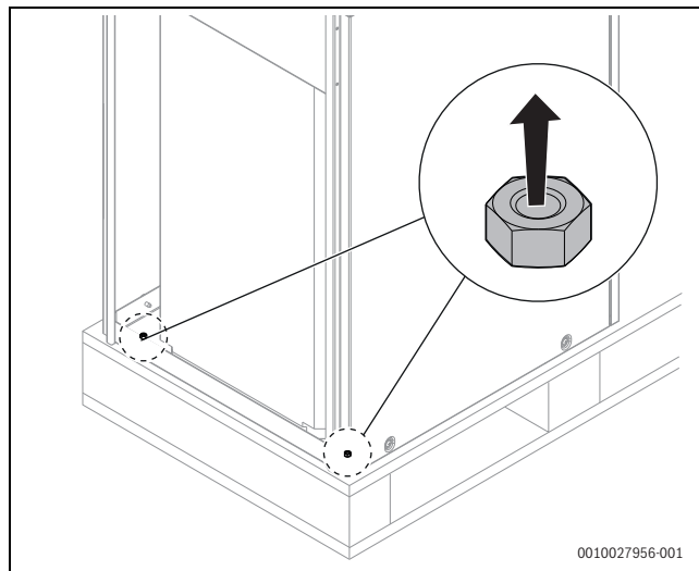
Fig. 46 Îndepărtarea siguranței de transport din partea din spate, jos, a rezervorului
