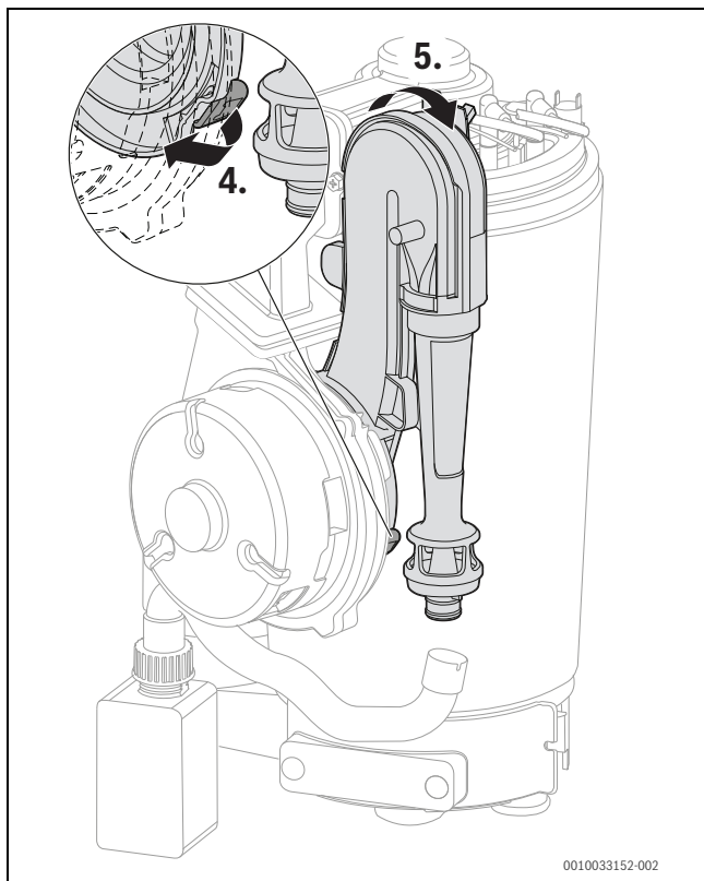
Fig. 115 Scoaterea țevii Venturi
