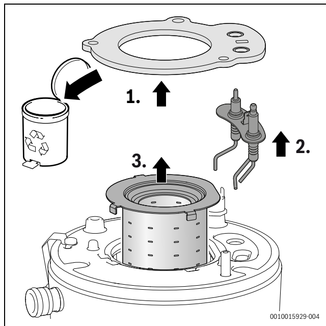
Fig. 120 Scoateți arzătorul
