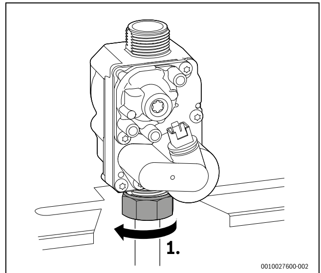
Fig. 137 Desfacerea piuliței oarbe
