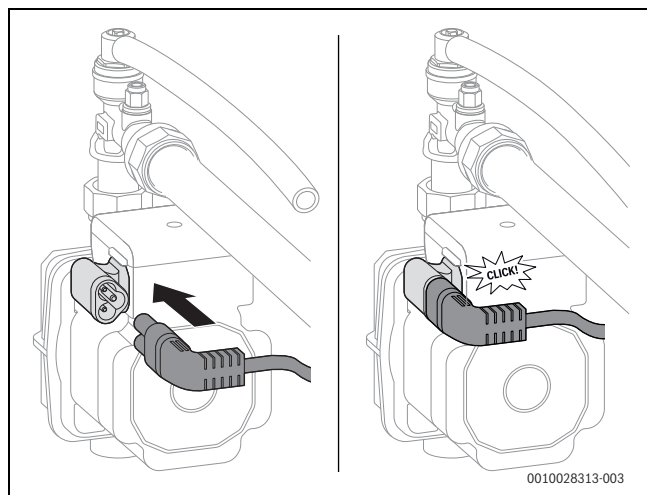
Fig. 84 Racordarea electrică a pompei de încărcare în straturi
