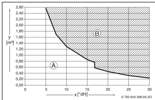
Fig. 40 Cerințe privind apa de alimentare și completare în °dH pentru aparate < 50 kW
