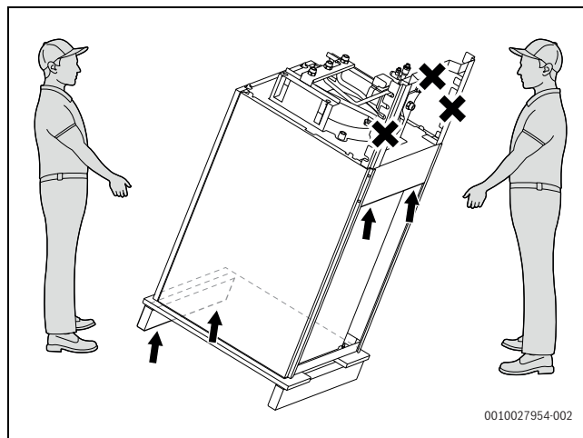
Fig. 45 Transportarea rezervorului
