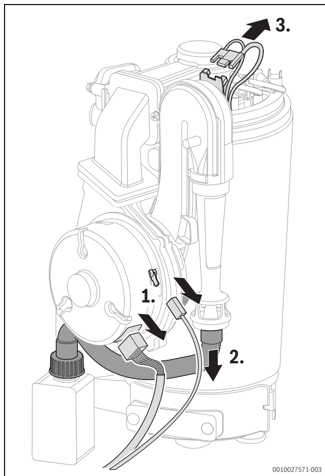
Fig. 114 Scoaterea steckerului și a furtunului de gaz
