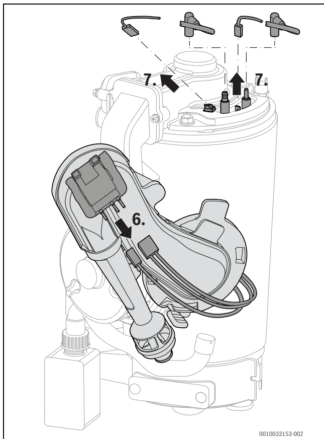
Fig. 116 Scoaterea cablului
