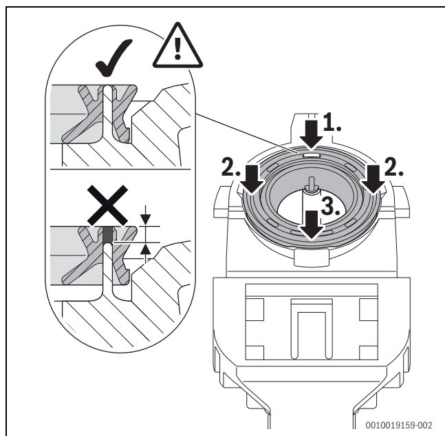
Fig. 146 Fixarea prin apăsare a garniturii de etanșare
