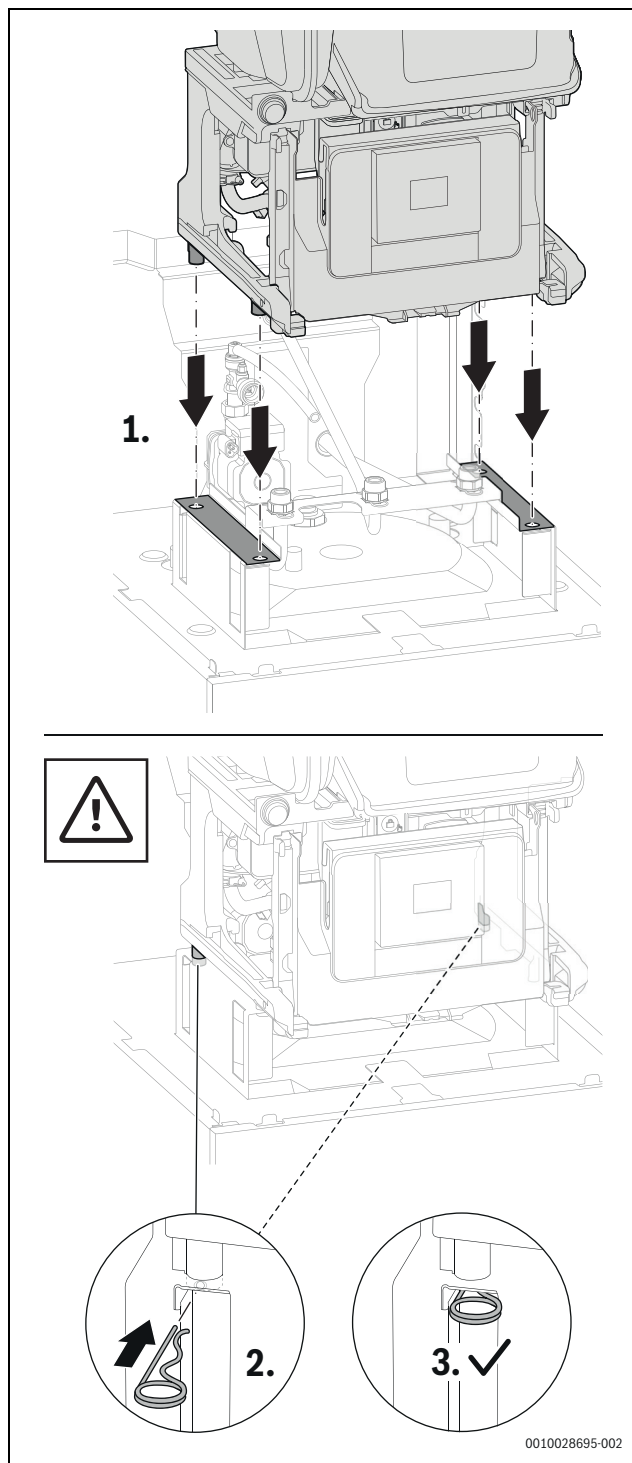
Fig. 54 Așezarea aparatul pe rezervor și fixarea cu 2 splinturi
