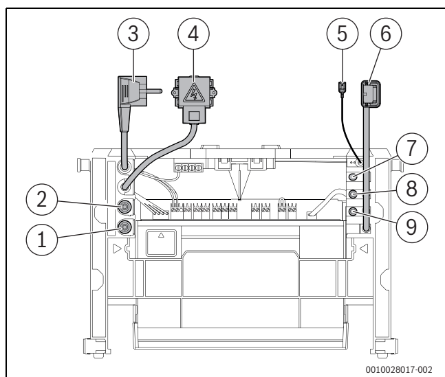
Fig. 79 Starea de livrare a dispozitivului de comandă cu componente conectate
