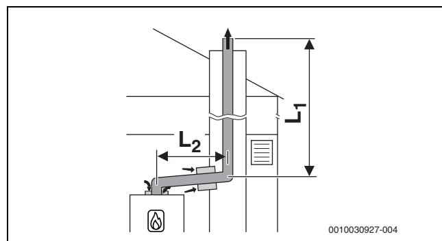
Fig. 31 Ghidarea rigidă a gazelor arse în puț conform B 53p cu alimentare cu aer dependentă de aerul din încălț la nivelul aparatului și elementului de legătură concentric dintre încăperea centralei termice și puț
