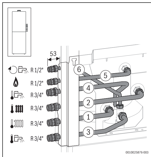
Fig. 12 Vedere din spate (dimensiuni în mm): accesorii CS 10 montate pe partea dreaptă
