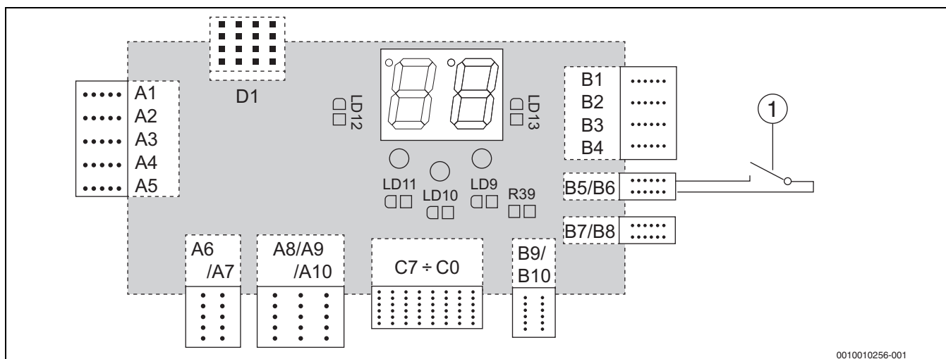
Fig. 23 Racord termostat de ambianță
