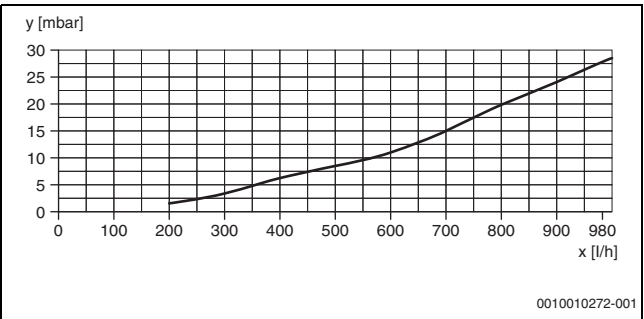
Fig. 37 Rezistență hidraulică Tronic Heat 3500 4...12 kW
