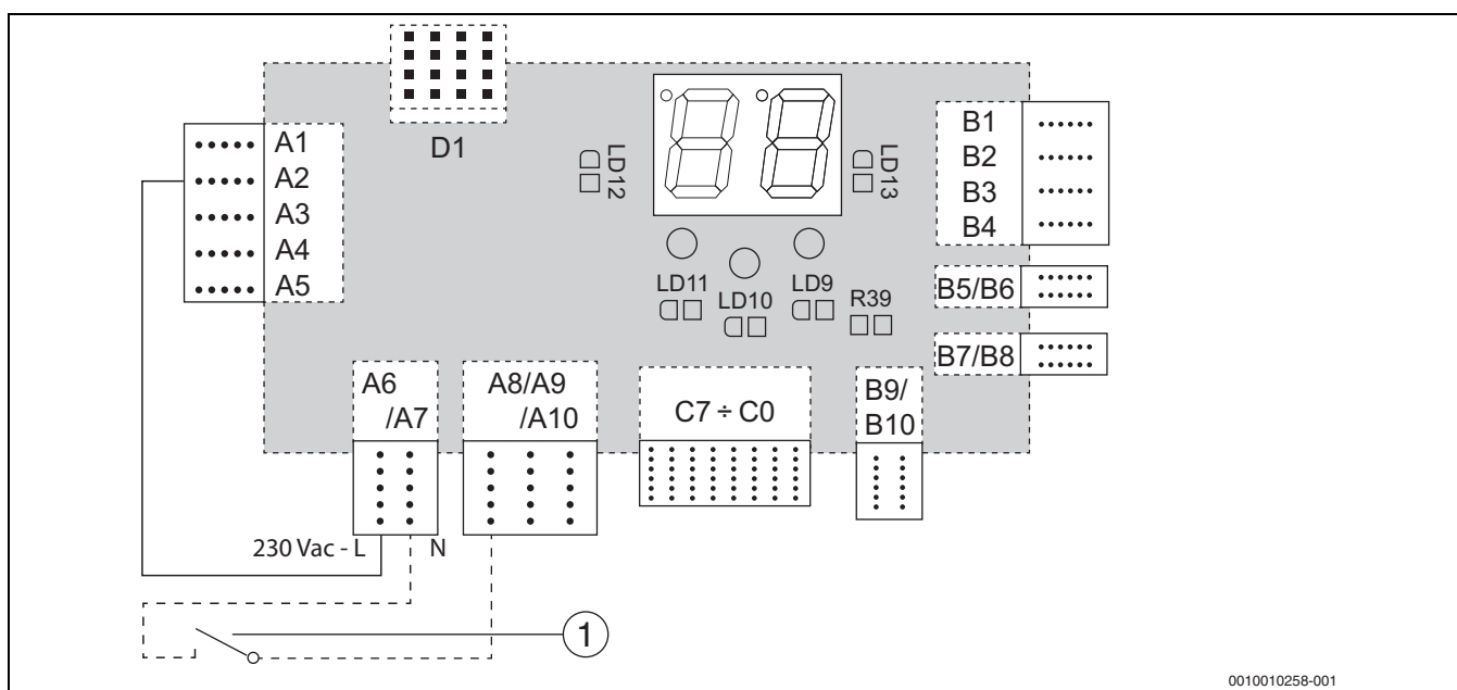
Fig. 24 Sistem de comandă al cazanului de încălzire prin intermediul comenzii căldurii de la distanță (conductor neutru)
