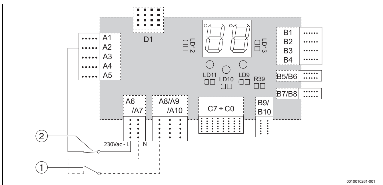
Fig. 26 Blocarea cazanului de încălzire și a sistemului de comandă prin intermediul comenzii căldurii de la distanță (conductor neutru)
