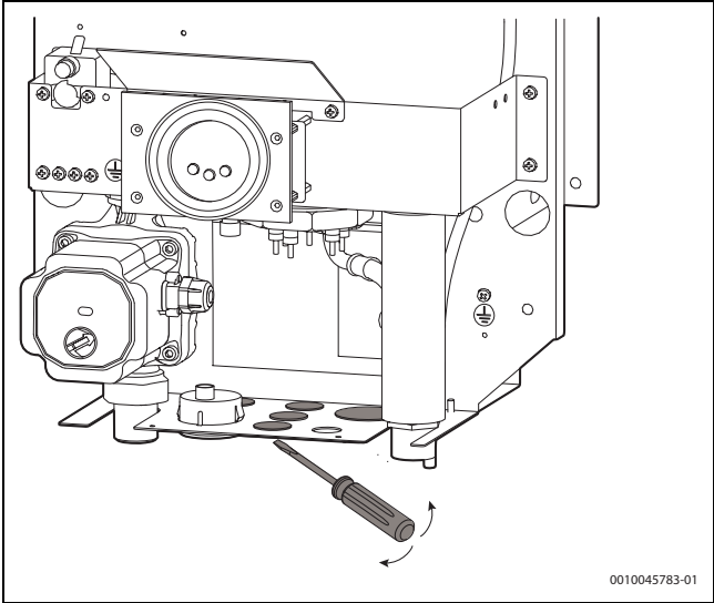
Fig. 16 Montarea orificiilor de trecere 1
