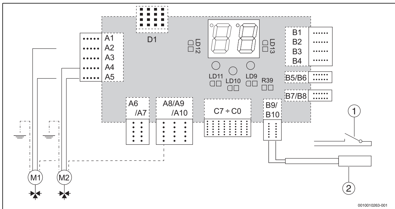
Fig. 30 Sistem de comandă al încălzirii apei calde (WW) prin intermediul senzorului de temperatură sau al contactului termostatului de apă caldă
