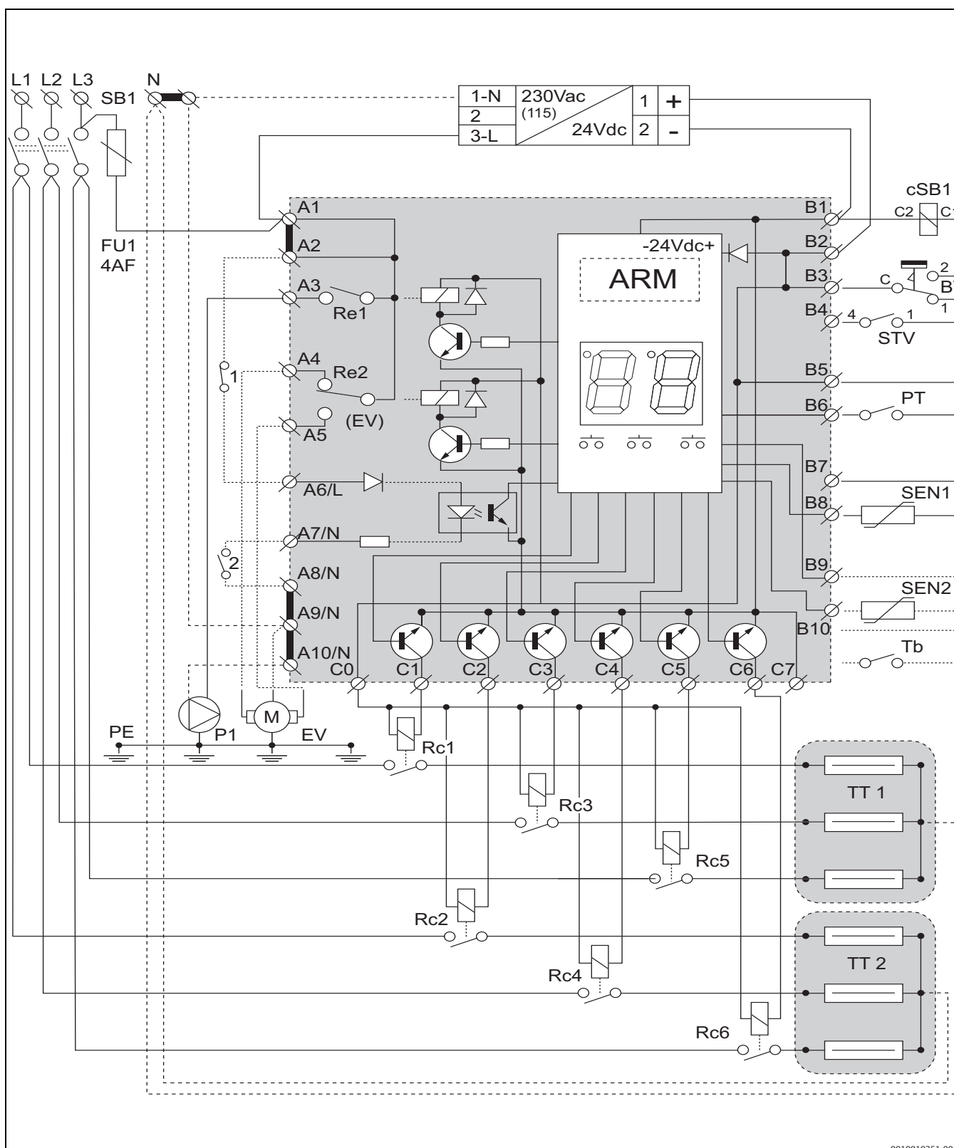
Fig. 21 Schema de utilizare a cazanului de încălzire Tronic Heat 3500 (15-24 kW), 3x 400/230 V AC
