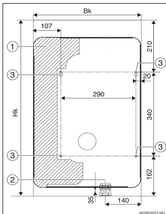
Fig. 9 Dimensiuni ale orificiilor pentru fixarea cazanului de încălzire pe perete și pentru cablul de alimentare al cazanului de încălzire Tronic Heat 3500 15-24 kW
