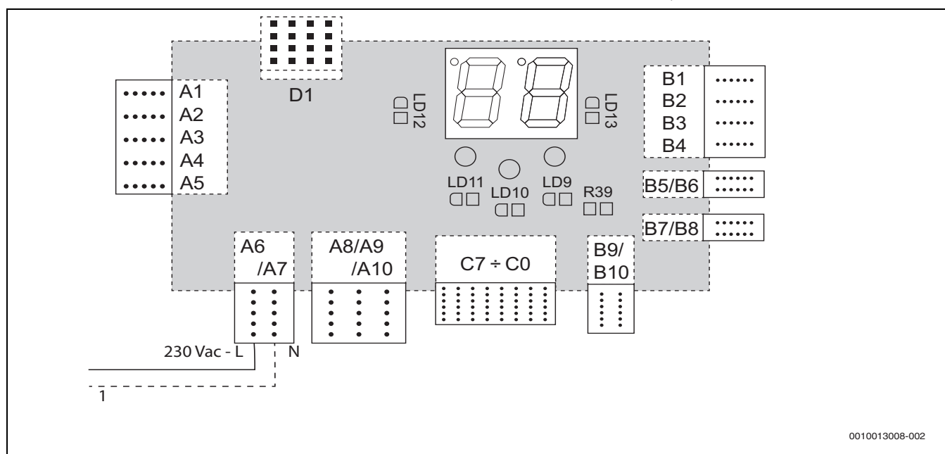
Fig. 28 Sistem de comandă al cazanului de încălzire prin intermediul comenzii căldurii de la distanță (tensiune externă)
