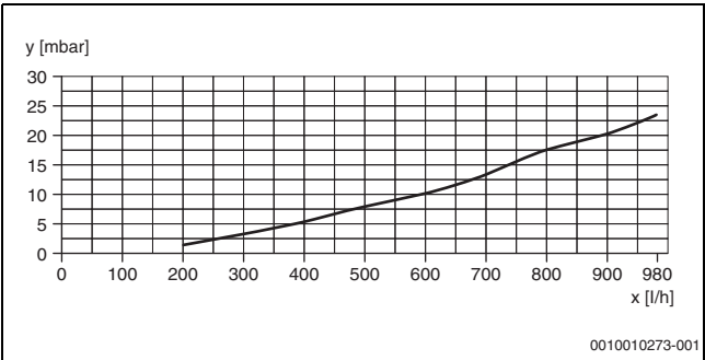
Fig. 38 Rezistență hidraulică Tronic Heat 3500 15...24 kW
