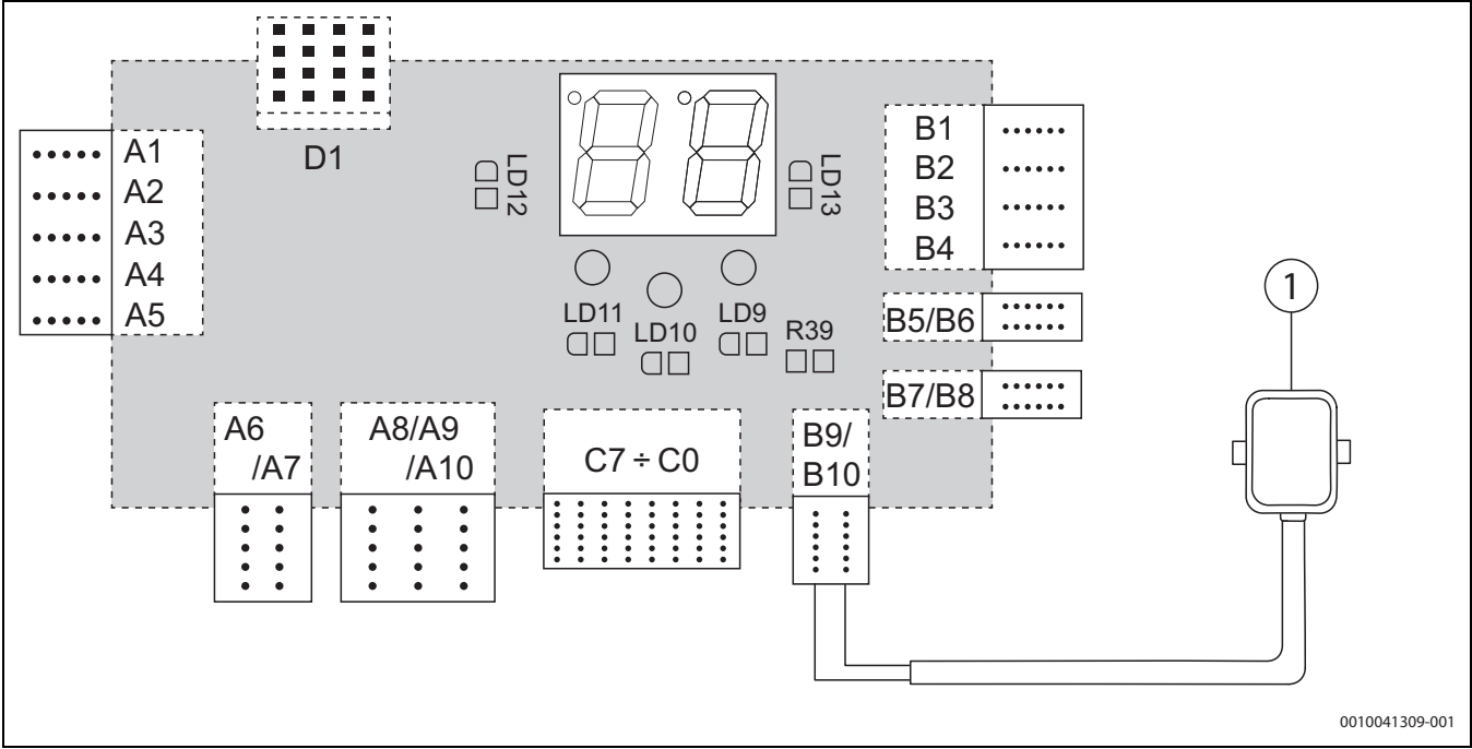
Fig. 33 Conectarea la un senzor de temperatură exterioară pentru control echitermic
