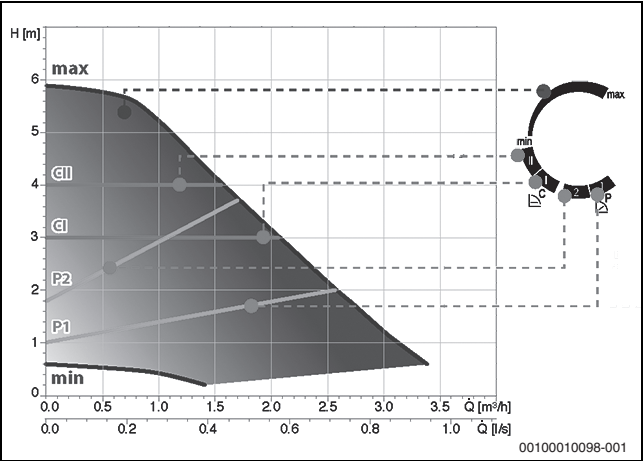
Fig. 36 Înălțimea de sarcină a pompei circuitului de încălzire pentru cazanul de încălzire Tronic Heat 3500 4...24 kW
