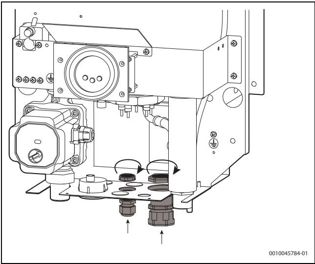
Fig. 17 Montarea orificiilor de trecere 2
