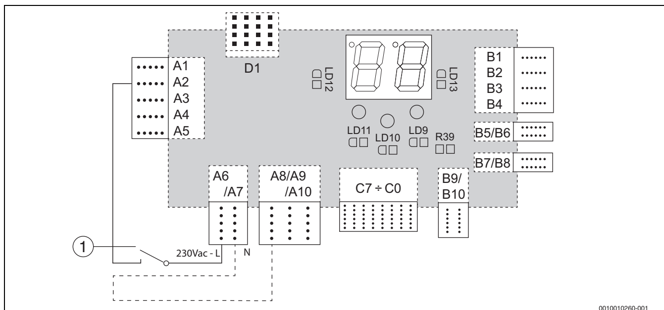
Fig. 25 Sistem de comandă al cazanului de încălzire prin intermediul comenzii căldurii de la distanță (conductor de fază)
