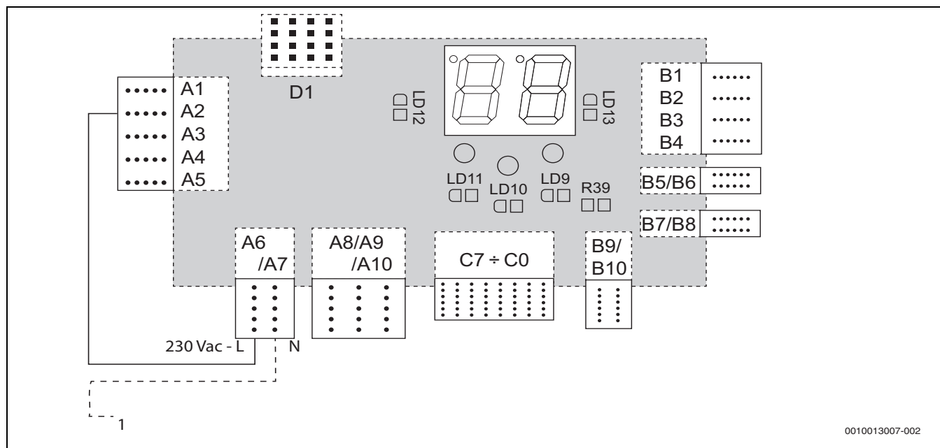
Fig. 27 Sistem de comandă al cazanului de încălzire prin intermediul comenzii căldurii de la distanță (conductor neutru extern separat, contact comutat liber de tensiune)
