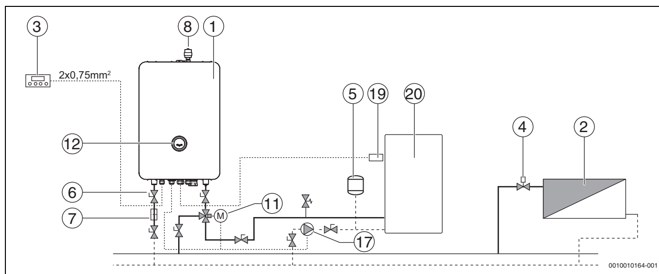
Fig. 41 Exemplu pentru racordul cazanului de încălzire electric Tronic Heat 3500 ca sursă de căldură de rezervă
