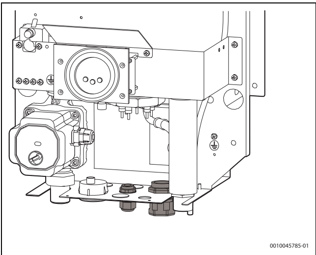
Fig. 18 Montarea orificiilor de trecere 3
