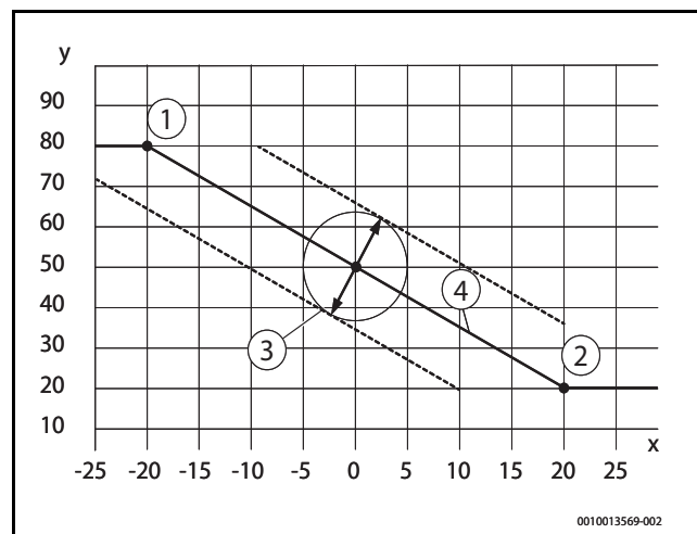
Fig. 35 Curbă de încălzire în funcție de temperatura exterioră
