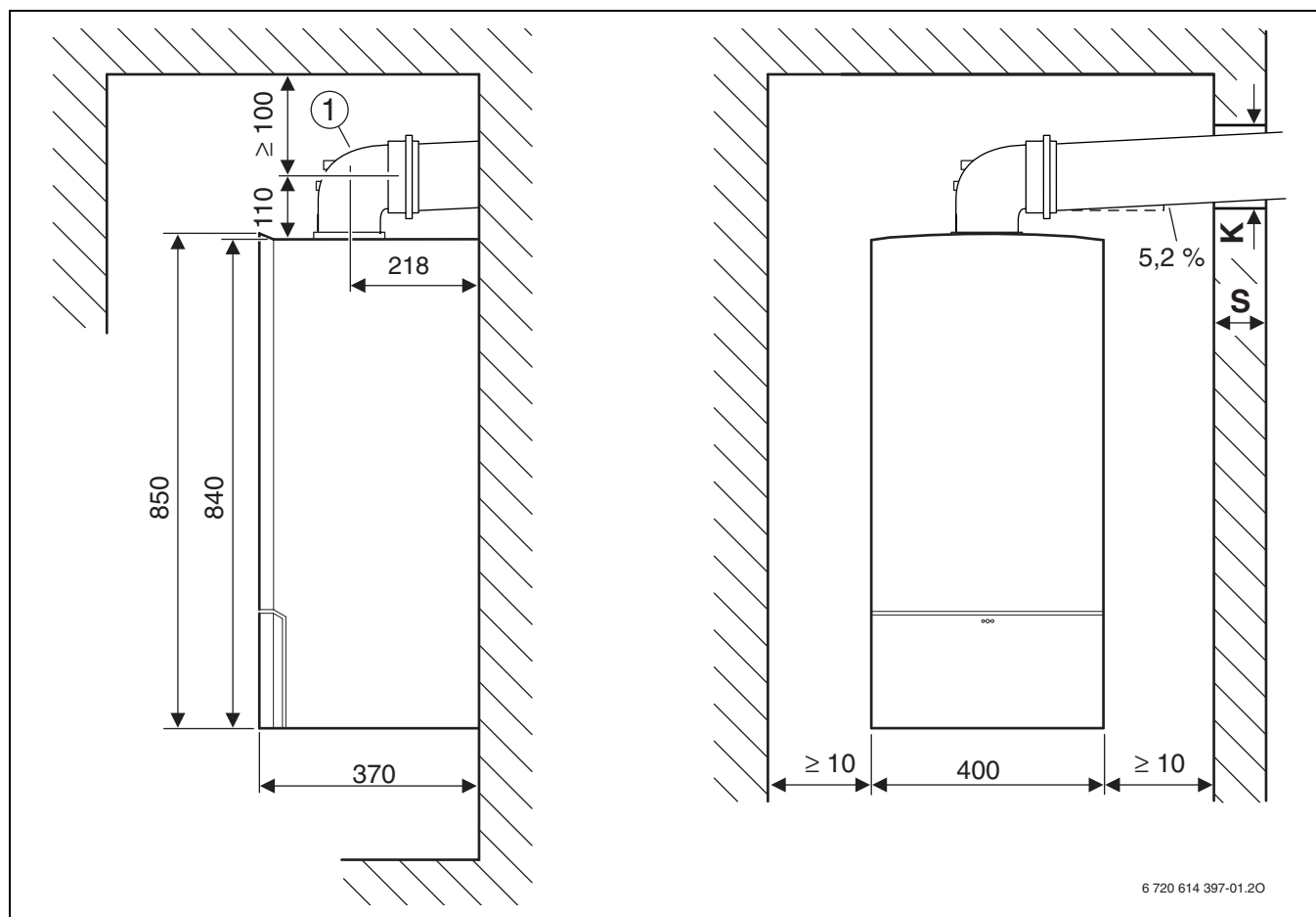
Fig. 5 unei conducte de gaze arse Ø 80/125 mm sau Ø 80 mm
