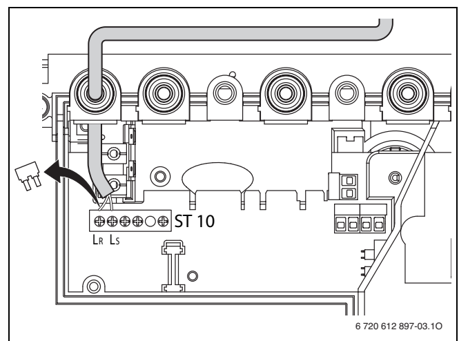
Fig. 19 Racord (AC 230 V, îndepărtați puntea între L_S și L_R )
