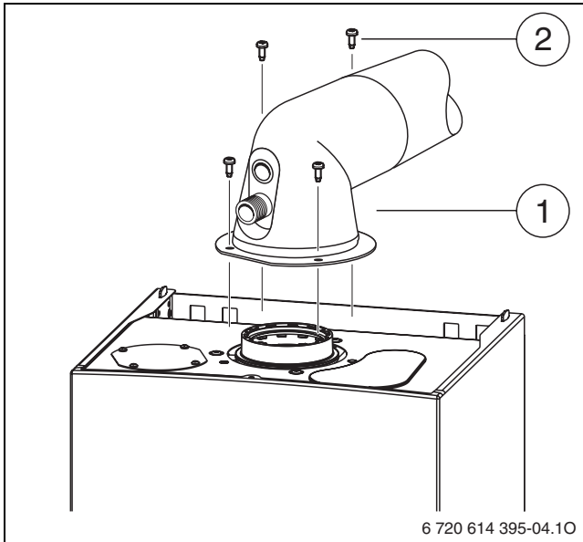
Fig. 14 Fixarea accesoriilor pentru gaze arse
