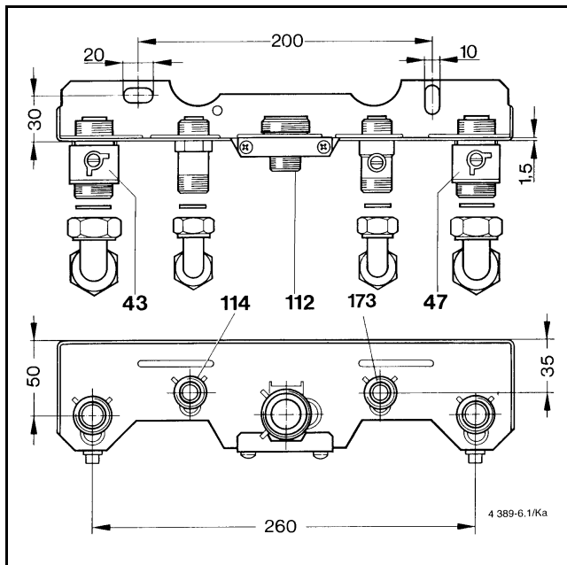
Fig. 7 Placă verticală de conexiune pentru montaj Nr. 492
