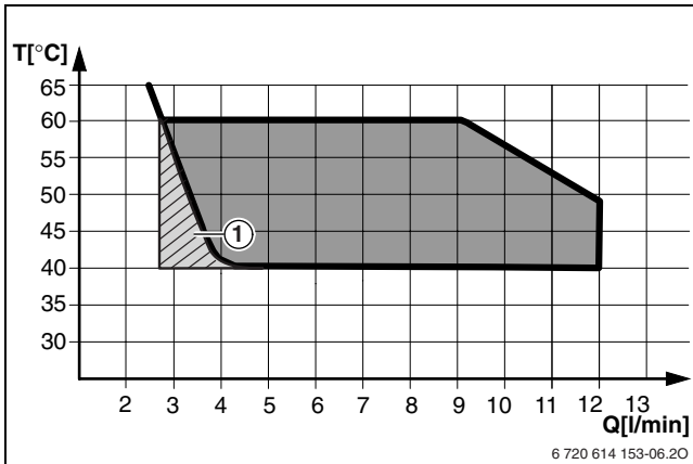
Fig. 29 Diagramă pentru o temperatură de intrare a apei reci de +15 °C
