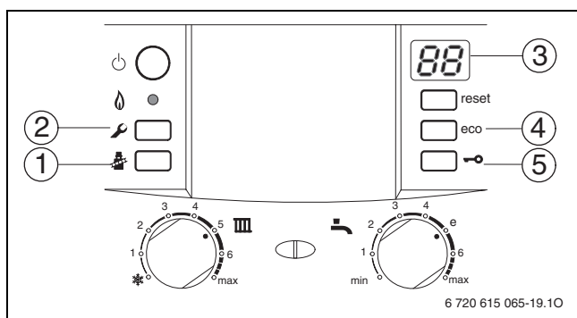
Fig. 36 Privire de ansamblu asupra elementelor de deservire
