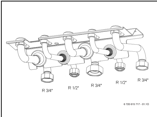
Fig. 6 Piesă verticală de legătură Nr. 1421
