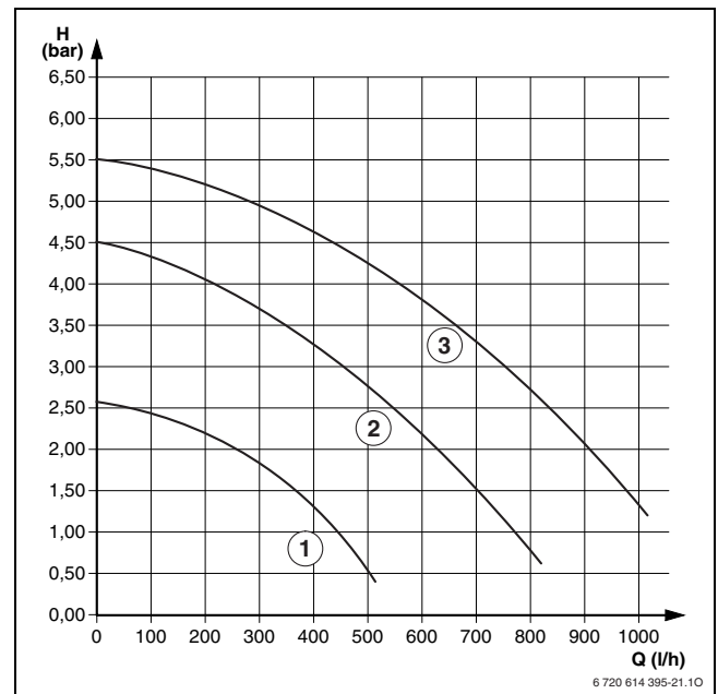
Fig. 35 Linii caracteristice (fără placă de racord a montajului)
