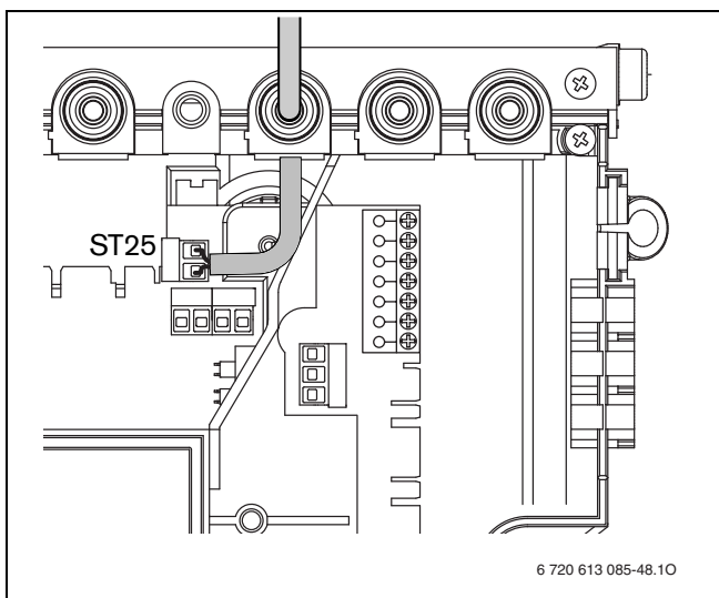
Fig. 22 Racord pompă de circulație
