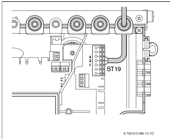
Fig. 20 Conectarea regulatorului de 24 V
