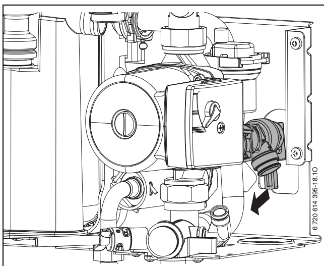
Fig. 58 Supapă de siguranță (încălzire)
