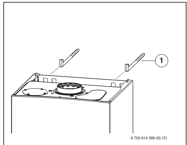
Fig. 9 Agățarea aparatului
