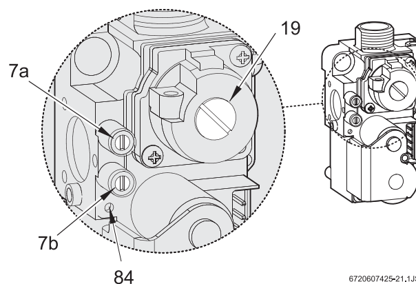
Fig. 4 Vană gaz
