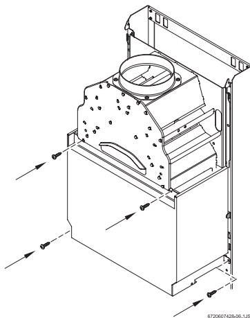
Fig. 1 Capac de protecție - KE
